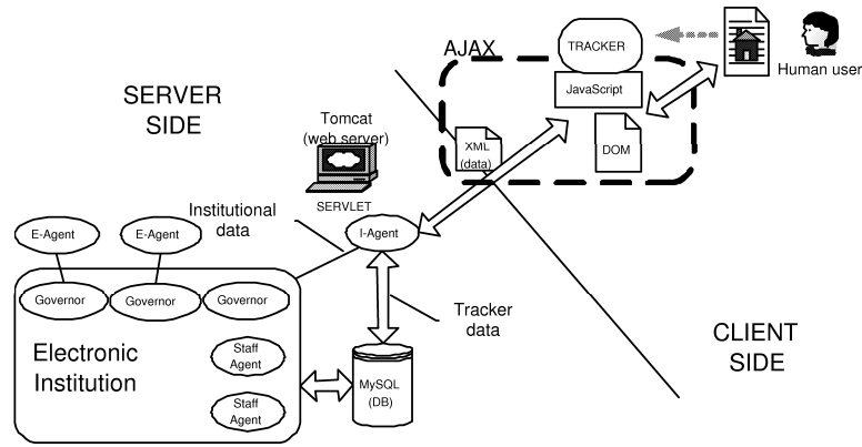
Fig. 4. Human - eI interaction
